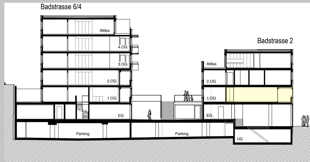
Querschnitt Badstrasse 6/4/2
