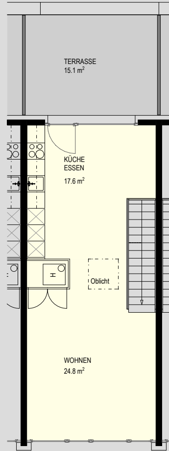
3. Obergeschoss
