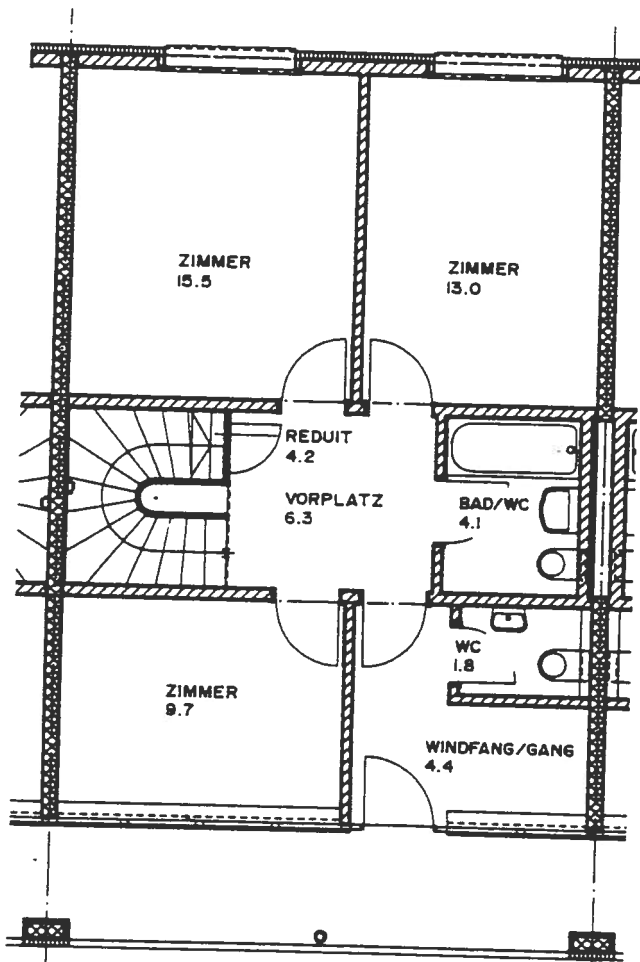
2. OBERGESCHOSS
