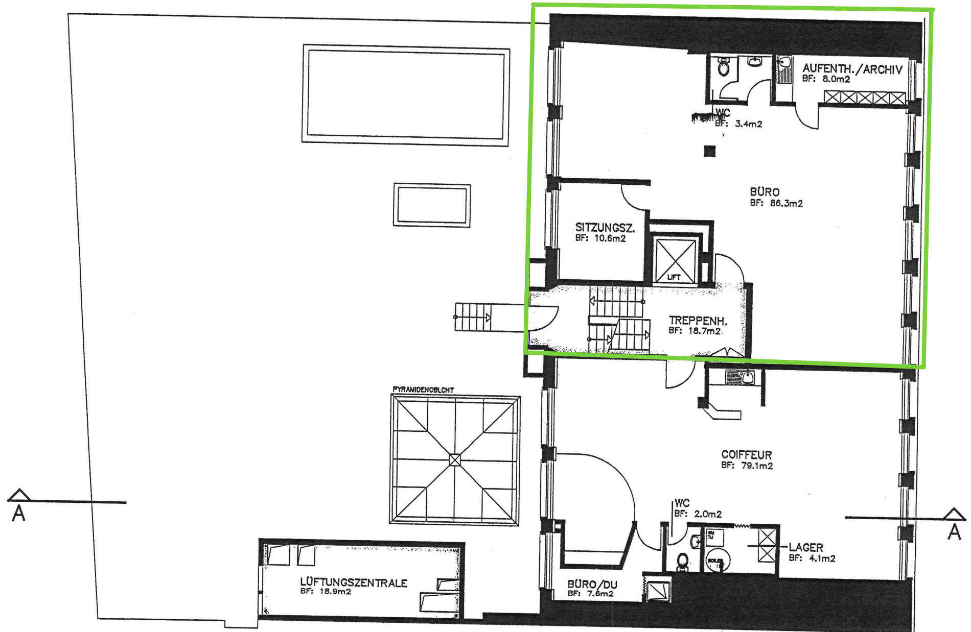
1. OBERGESCHOSS
