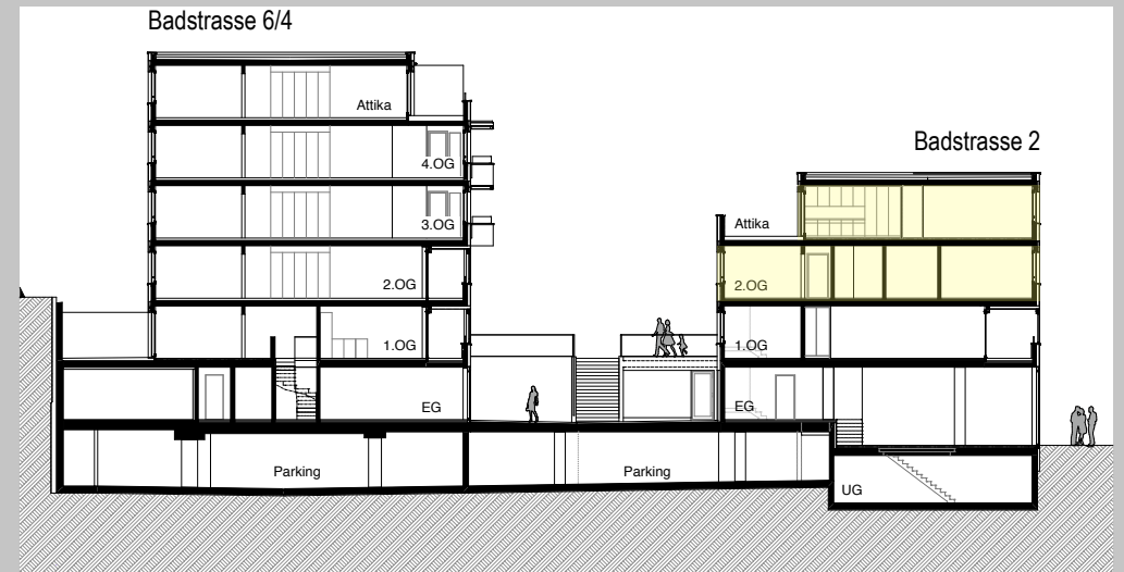
Querschnitt Badstrasse 6/4/2
