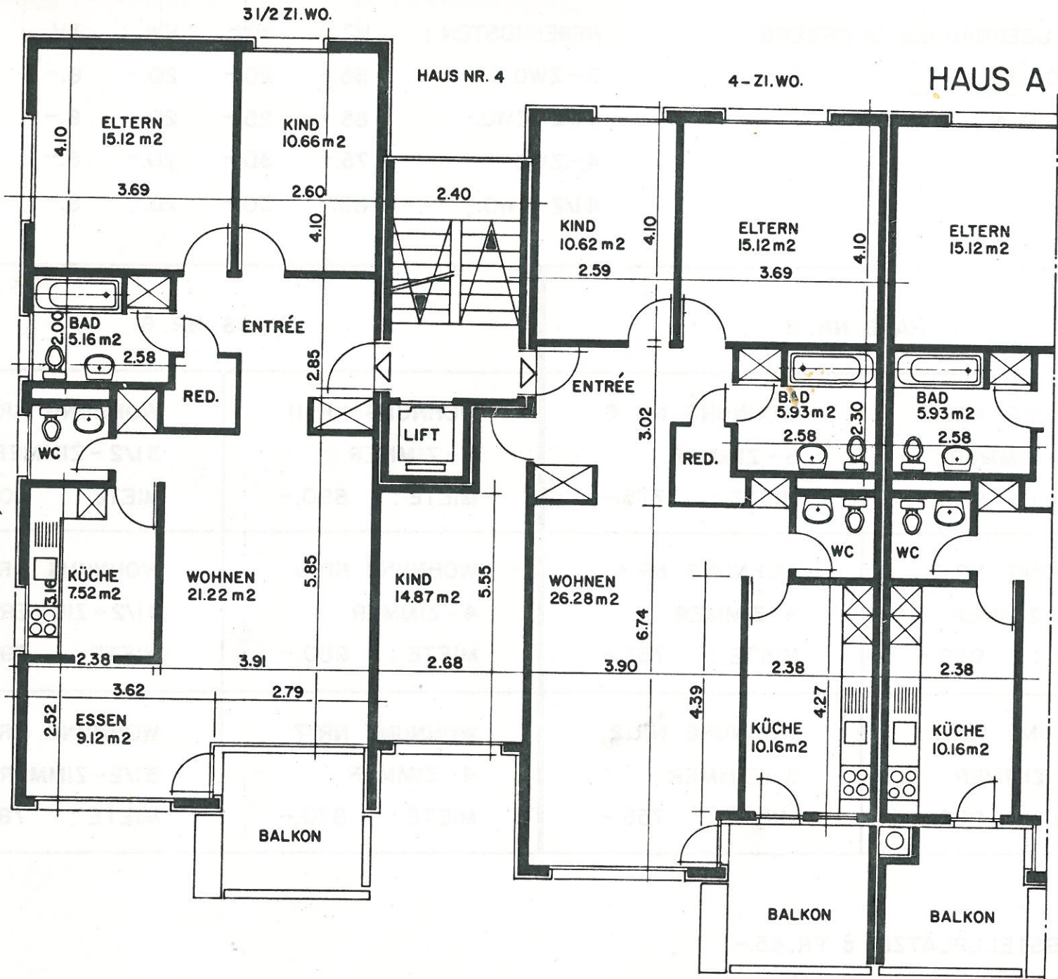
1.-4. OBERGESCHOSS
