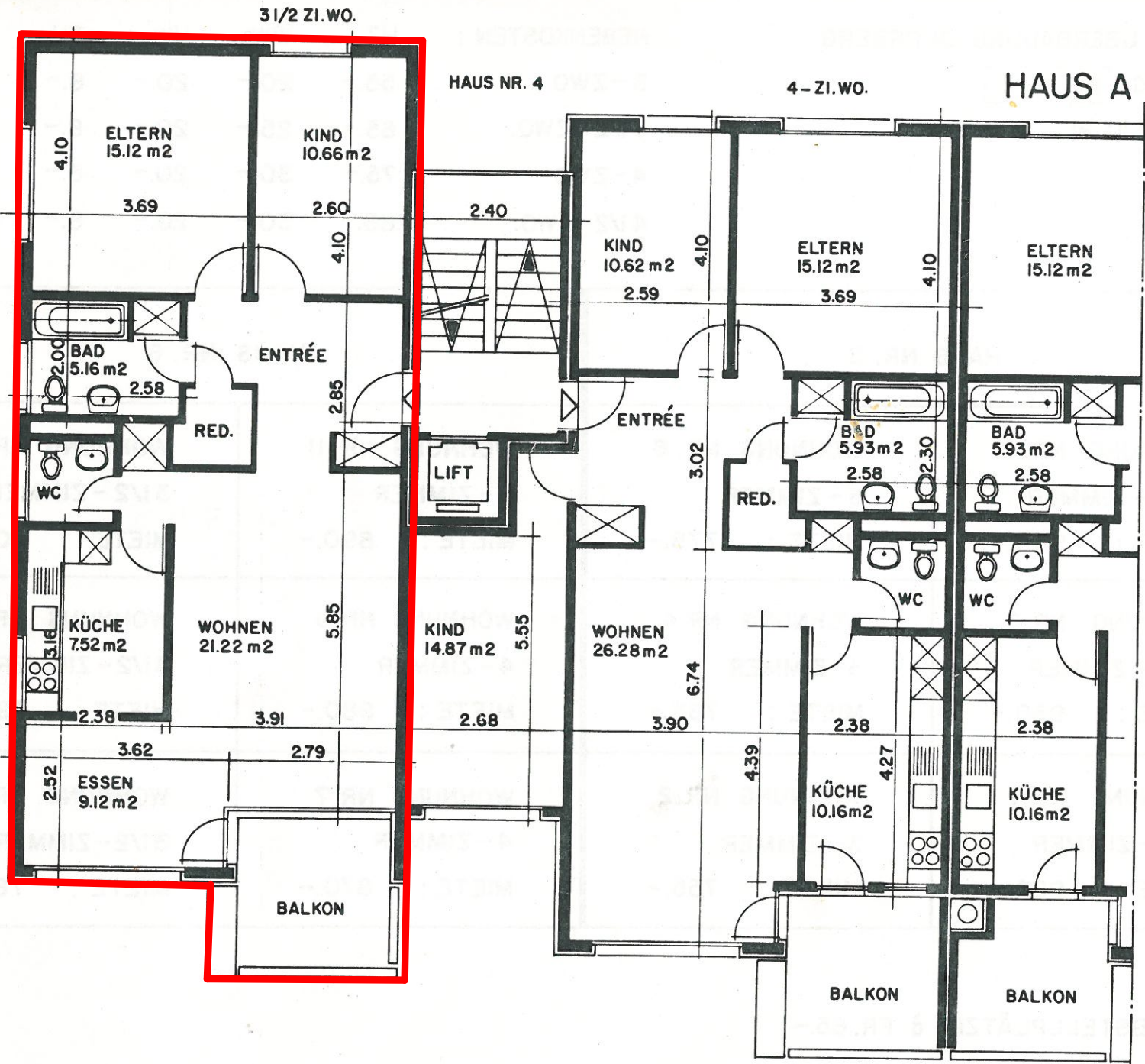
1.-4. OBERGESCHOSS
